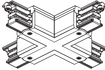
X-Baęlantı / X-connector
